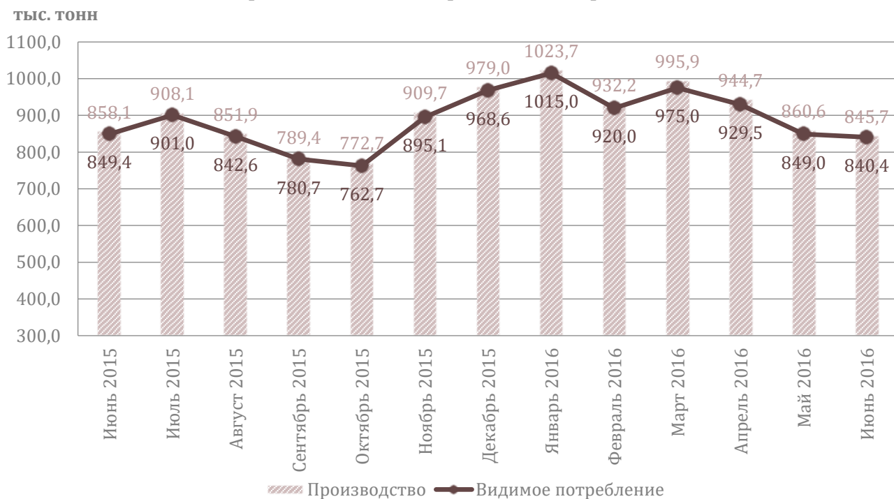
Рисунок 1 Динамика производства-потребления серной кислоты в РФ –2015-2016 гг., тыс. тонн.
